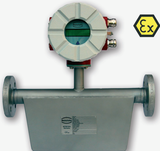
מד זרימה קוריאוליס ■
